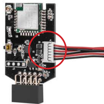
内附电源 / 重置 / Speaker Y 线
