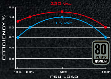
80 PLUS钛金牌认证的超高效率设计，有效节省电费与废热的产生。
