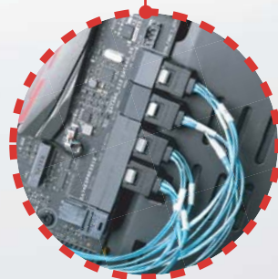
Connecter le CPS03-RE aux ports SATA de la carte mère
