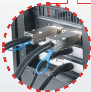
Connecter l'adaptateur Mini-SAS et les câbles externes de l'adaptateur secteur
