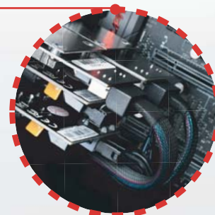
Mini-SASアダプタと電源アダプタの内部ケーブルを接続します
