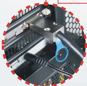
Collegare Mini-SAS SFF-8088 e l'adattatore di alimentazione alla memoria esterna
